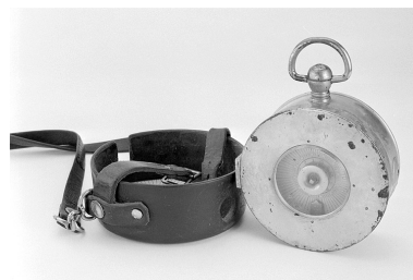
Le contrôleur hors de son étui. Le disque de papier, visible derrière le cadran vitré, permet l'enregistrement des heures de passage. Phot. Jérôme Mongreville IVR43_20022501006X
