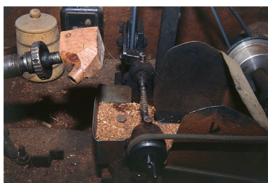
Partie gauche : détail du support de l'ébauchon. A droite, arbre cranté horizontal faisant office de fraise. Phot. Jérôme Mongreville IVR43_20003901024ZA
