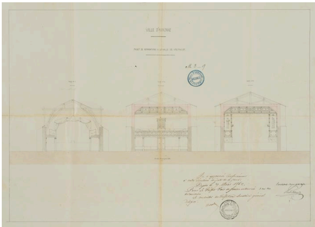
Ville d'Auxonne. Projets de réparations à la salle de spectacle. [Coupe transversale]. 3 mai 1842.
