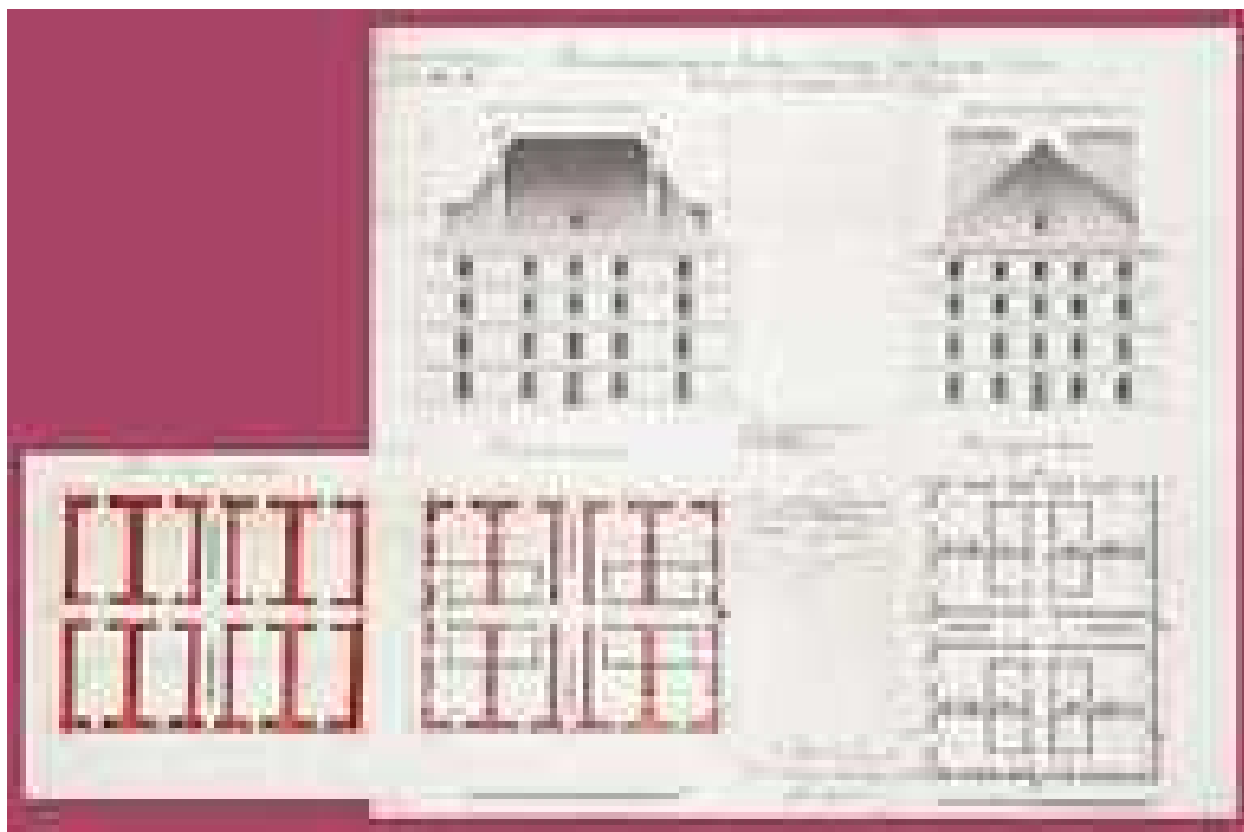
Elévation et plans des caves, du rez-de-chaussée et du premier étage du corps de casernes à construire. Dessin aquarellé : 50,5 x 55,5 cm, 1738.
