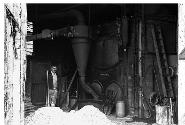
Chaudière Meunier et Cie. Phot. Laurent Poupard IVR43_19893900279Z
