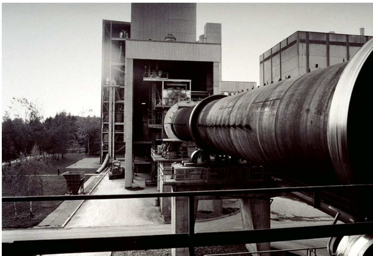
Four rotatif Polysius.
