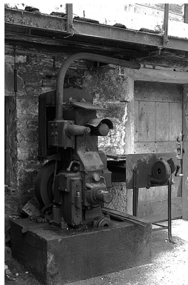
Moteur diesel Cérés. Phot. Laurent Poupard IVR43_19923901226Z
