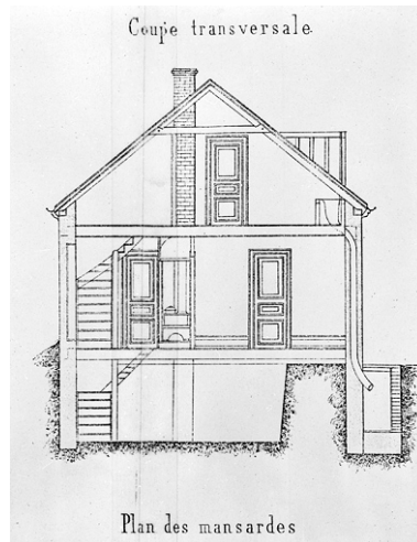
maison ouvrière, coupe transversale Phot. Yves Sancey IVR43_19829000331V
