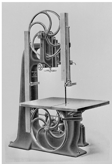
Scie à ruban à table inclinable. Phot. Yves Sancey IVR43_20022500920X
