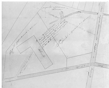
Plan-masse de l'usine. Phot. Jérôme Mongreville IVR43_20019000239X
