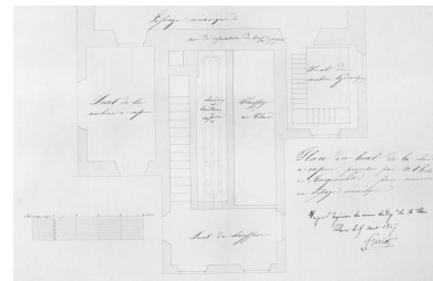
Plan du local de la chaudière à vapeur projetée par M. Erhard à Rougemont pour mouvoir un tissage mécanique. Phot. Jérôme Mongreville IVR43_20019000255X
