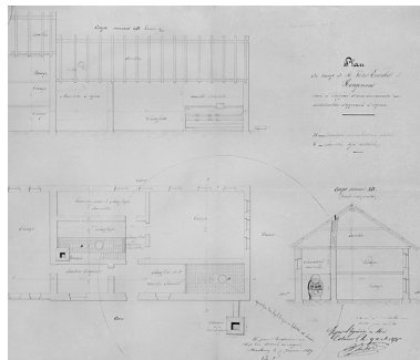
Plan du tissage de M. Victor Erhard à Rougemont dressé à l'appui d'une demande en autorisation d'appareils à vapeur. Phot. Jérôme Mongreville IVR43_20019000027V
