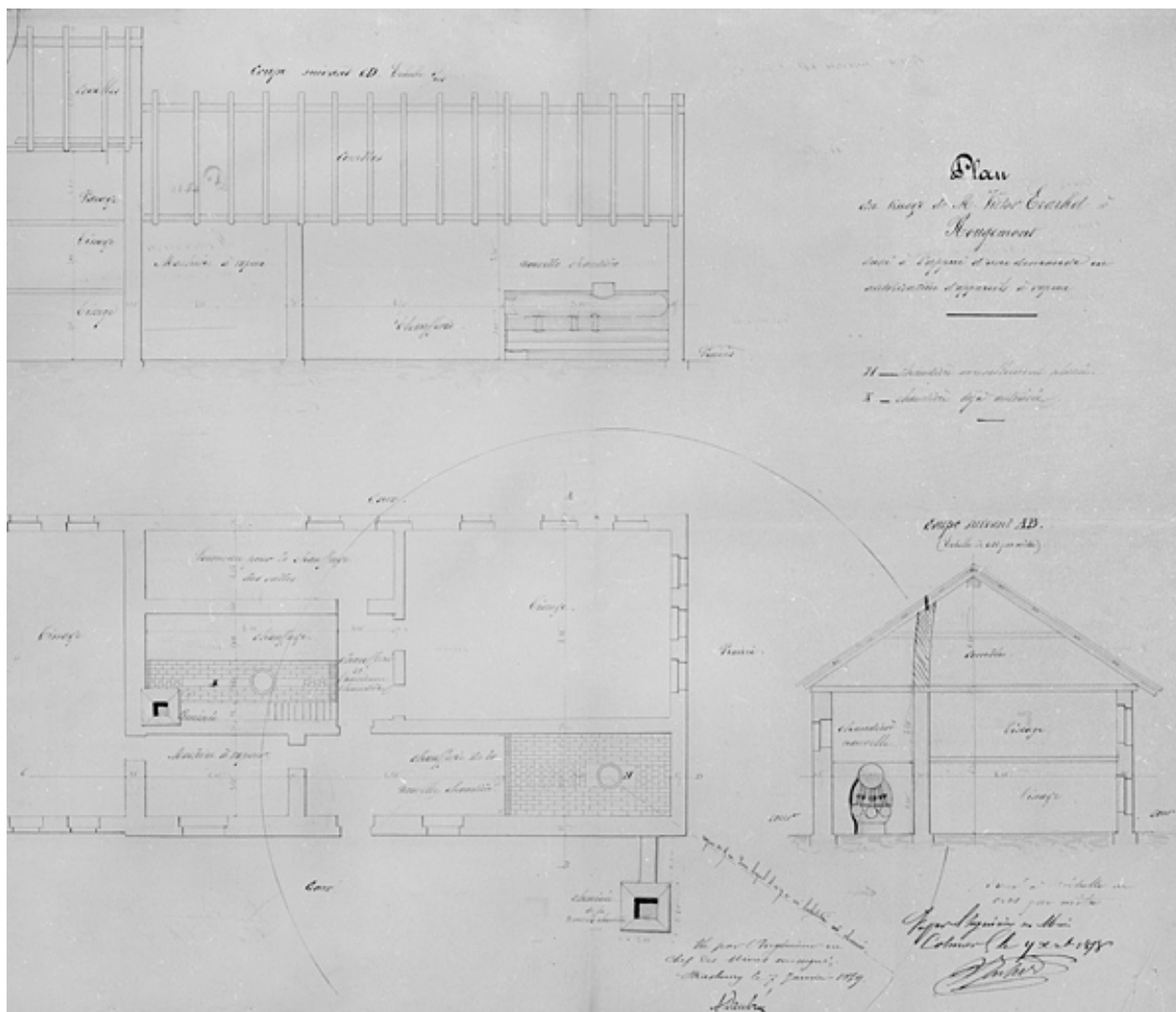
Plan du tissage de M. Victor Erhard à Rougemont dressé à l'appui d'une demande en autorisation d'appareils à vapeur.
