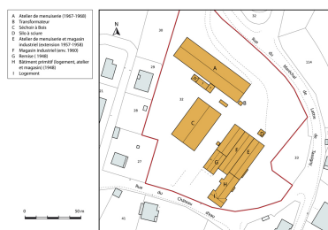
Plan-masse et de situation, section AB. Dess. Mathias Papigny IVR43_20142501917NUDA
