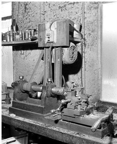
Vue d'ensemble, avec son moteur. Phot. Jérôme Mongreville IVR43_20003900990X
