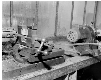
Mandrin porte-outils et chariot mobile. Phot. Jérôme Mongreville IVR43_20003900998X
