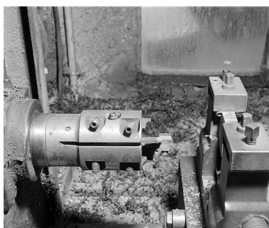
Détail du mandrin porte-outils. Phot. Jérôme Mongreville IVR43_20003901000X
