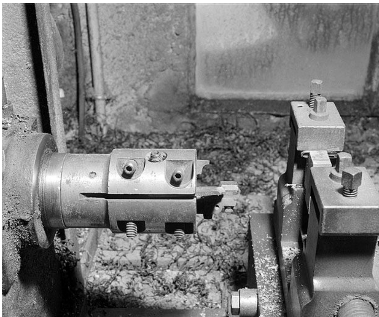
Détail du mandrin porte-outils.
