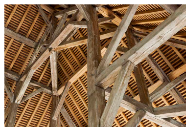
Croupe du séchoir. Partie supérieure de la charpente. Phot. Jérôme Mongreville IVR43_20162501142NUC4A
