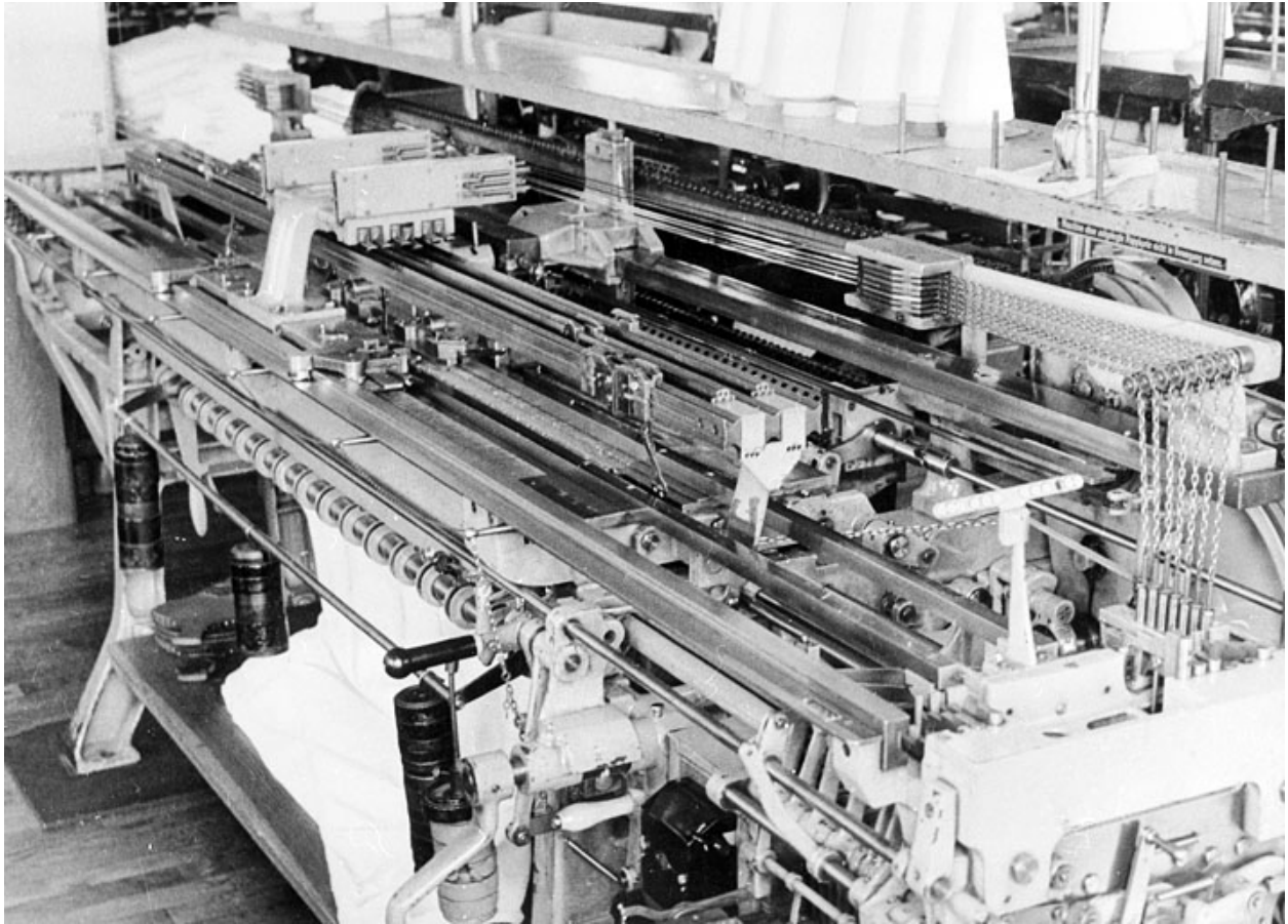
Machine à tricoter en panneau (marque Stoll, type Lifado).
