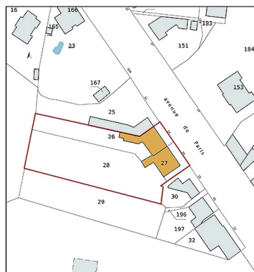
Plan-masse et de situation, extrait du plan cadastral (2021). Dess. Pierre-Marie Barbe-Richaud IVR26_20215800059NUDA
