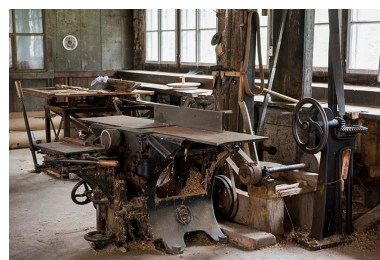
Usine : raboteuse Muller et commande de la turbine Laurioz. Phot. Sonia Dourlot IVR43_20172500030NUC4A
