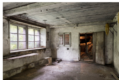
Usine : salle au 1er étage de soubassement, donnant sur la chambre d'eau. Phot. Sonia Dourlot IVR43_20172500025NUC4A
