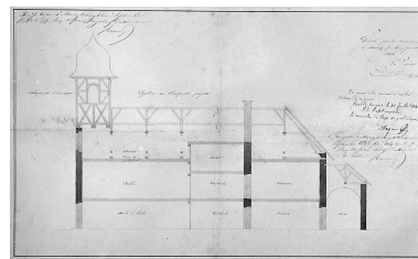
[Coupe de l'ancienne église montrant la charpente projetée], 1843. Phot. Jérôme Mongreville, Autr. Vital Ponard IVR43_19953900058X
