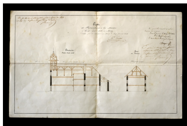
Projet de réparations à la maison d'école de la ville de Morez. Elévation de la maison d'école actuel [et] Coupe en travers, 1843. Phot. Yves Sancey, Autr. Vital Ponard IVR43_20103900027NUC2A
