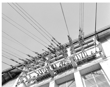
Détail du transformateur : départ de fils électriques (cadrage vertical).
