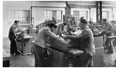
Machine à rectifier de haute précision. Phot. Yves Sancey IVR43_20009000873X
