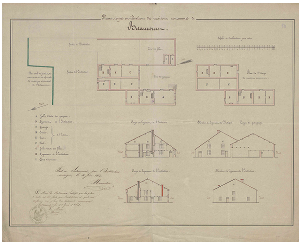
Plans, coupes et élévations des maisons communes de Betaucourt. Fait par l'instituteur le 10 juin 1864.
