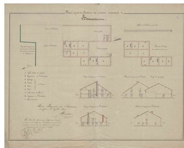
Plans, coupes et élévations des maisons communes de Betaucourt. Fait par l'instituteur le 10 juin 1864. Phot. Sonia Dourlot
