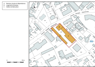
Plan-masse et de situation. Extrait du plan cadastral, 2019. Dess. Bertrand Turina IVR43_20192501123NUDA
