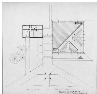
Plan du sous-sol, 1958.
