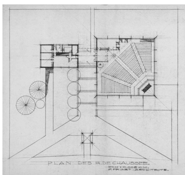
Plan du rez-de-chaussée, 1958.
