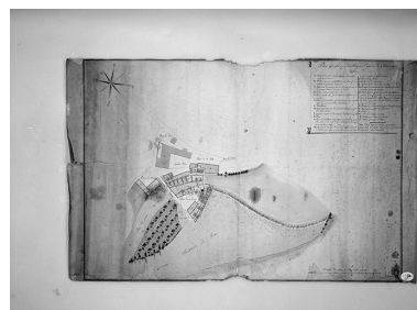
Plan géométrique des forges et usines de Chenecey, s.d. [début 19e siècle]. Phot. Yves Sancey IVR43_19792501073V
