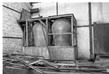
Atelier de galvanisation. Récipients en grès de 2000 litres (1979).
