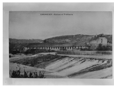
Chenecey (Doubs) - Les Forges, carte postale, s.d. [fin 19e ou début 20e siècle]. Phot. Yves Sancey IVR43_19792501062V
