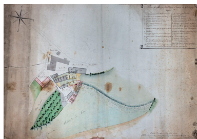
Plan géométrique des forges et usines de Chenecey, s.d. [milieu 19e siècle]. Phot. Jérôme Mongreville IVR43_20182500110NUC4A
