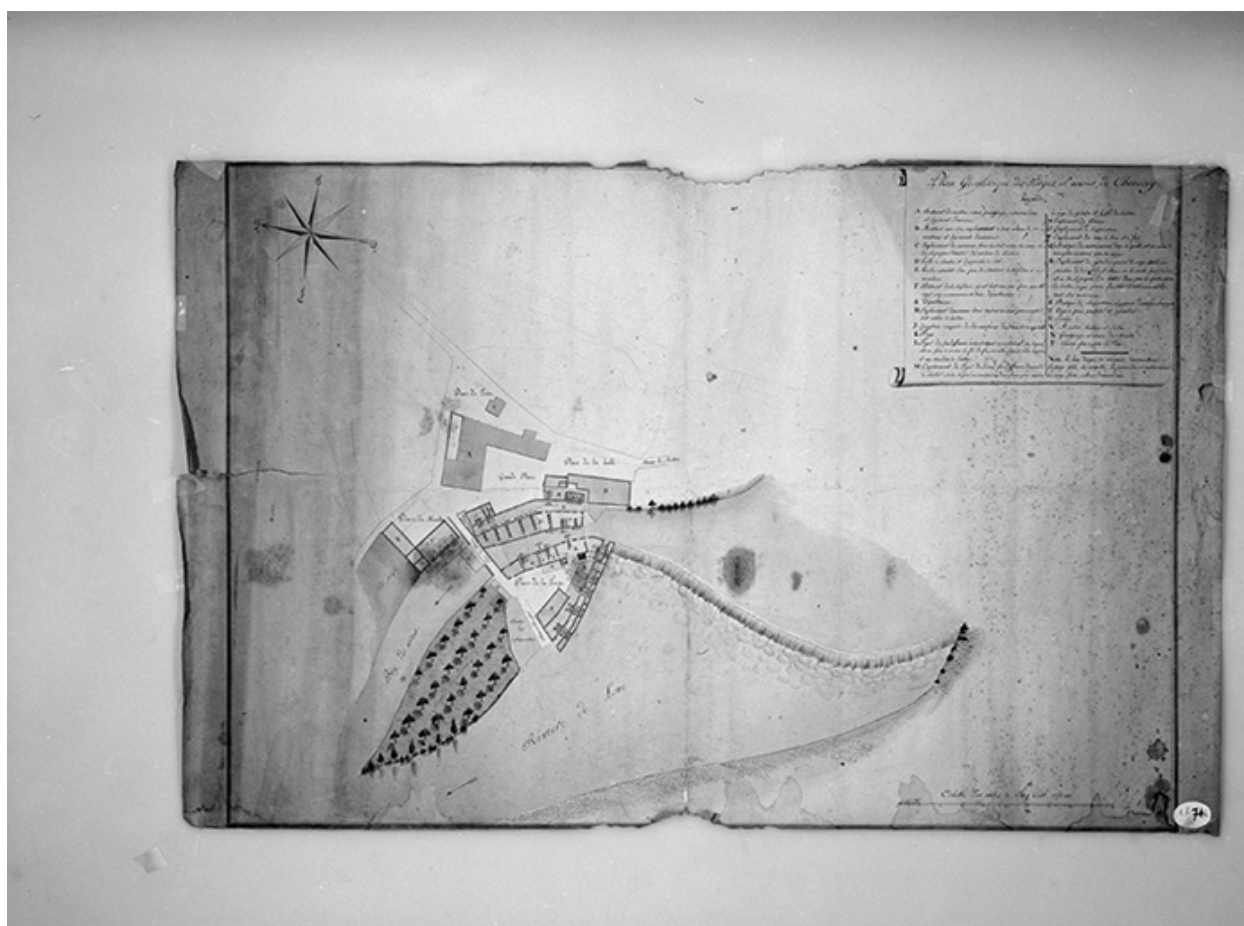
Plan géométrique des forges et usines de Chenecey, s.d. [début 19e siècle].
