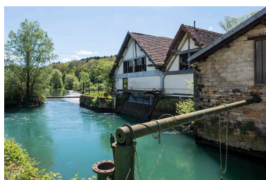
Pignons des ateliers et prise d'eau d'une turbine hydraulique. Phot. Jérôme Mongreville IVR43_20172500617NUC4A
