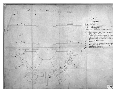
Dessin d'une roue hydraulique, s.d. [milieu 19e siècle]. Phot. Yves Sancey IVR43_19792501168V
