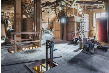
Etage de comble. Vue d'ensemble : monte-sac, chambres à grains. Phot. Jérôme Mongreville IVR43_20142501318NUC4A
