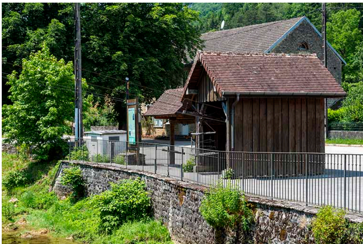
2020. Vue du transporteur automatique par câbles, de trois quarts droit.
