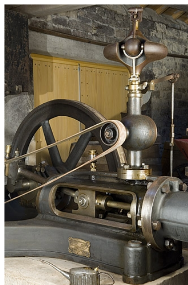
Machine à vapeur Diebold et Michel (Nancy). Détail. Phot. Jérôme Mongreville IVR43_20067000807NUCA
