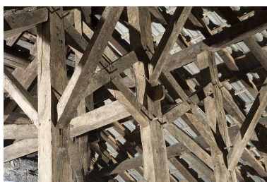
Charpente du fenil. Détail de partie haute. Phot. Jérôme Mongreville IVR43_20067000789NUCA
