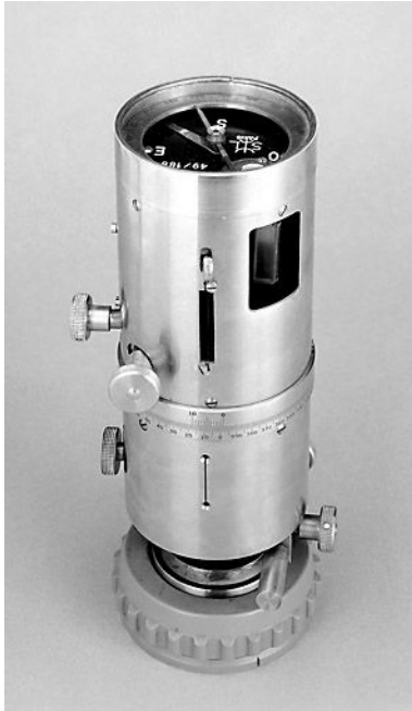
Vue d'ensemble d'un pantomètre.
