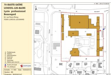
Plan-masse et de situation. Extrait du cadastre numérisé, 2011, section BE, échelle 1/ 1 500. Dess. André Céréza IVR43_20127000019NUDA
