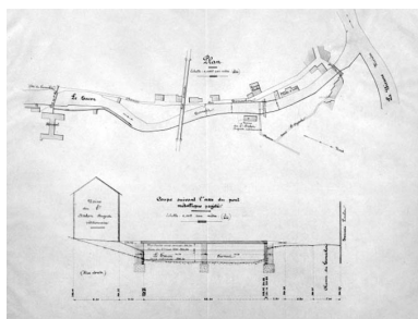
Construction d'une passerelle par le sieur Ardon (Auguste). Plan et profil. Phot. Jérôme Mongreville, (photographe) NEPASUTILISERMandrillon Phot. Messin IVR43_19943900420X
