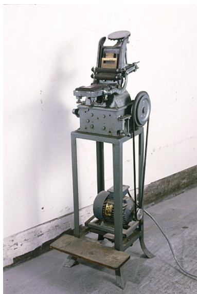
Vue d'ensemble. Phot. Jérôme Mongreville IVR43_20013900715ZA
