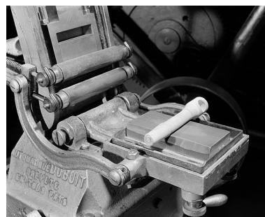
Détail : marbre, rouleaux encres et platine. Un élément de tire-bouchon est posé sur la platine. Phot. Jérôme Mongreville IVR43_20013900742X
