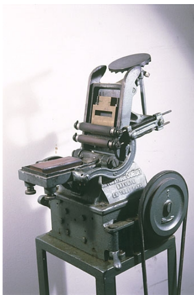
Vue rapprochée. De gauche à droite : platine, rouleaux encres, marbre et table d'encrage (soleil). Phot. Jérôme Mongreville IVR43_20013900717ZA
