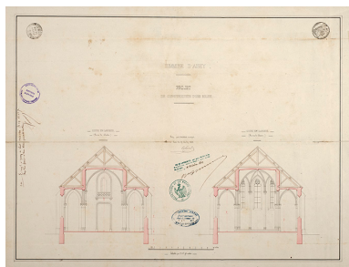
Projet de construction de l'église, coupe en largeur (1862). Phot. Jérôme Mongreville, Autr. Colard IVR43_20167000976NUC4A
