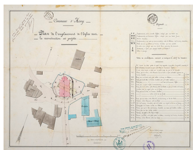
Projet de construction de l'église, plan projeté d'implantation du futur édifice (1862). Phot. Jérôme Mongreville, Autr. Colard IVR43_20167000977NUC4A
