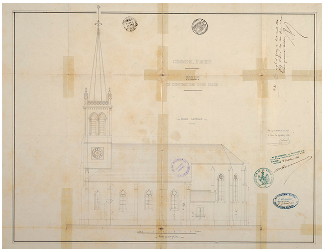
Projet de construction de l'église, façade latérale (1862).
