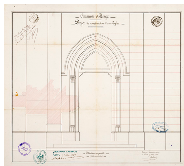
Projet de construction de l'église, élévation du portail (1862). Phot. Jérôme Mongreville, Autr. Colard IVR43_20167000971NUC4A
