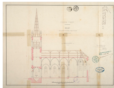
Projet de construction de l'église, coupe en longueur (1862). Phot. Jérôme Mongreville, Autr. Colard IVR43_20167000975NUC4A
