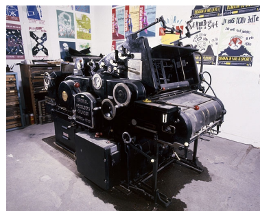
Vue d'ensemble de l'arrière de la machine. Phot. Jérôme Mongreville IVR43_20013900825XA
