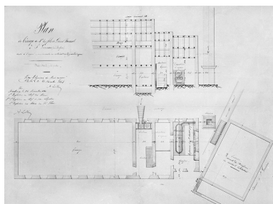
Plan du tissage de Mrs les fils de David Bumsel à Saint-Germain (près Belfort) dressé à l'appui d'une demande en autorisation d'appareils à vapeur. Phot. Jérôme Mongreville IVR43_20019000026V
