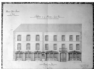
Dessin de la façade antérieure. Phot. Yves Sancey, Phot. Jules Laplanche IVR43_19927000270X
