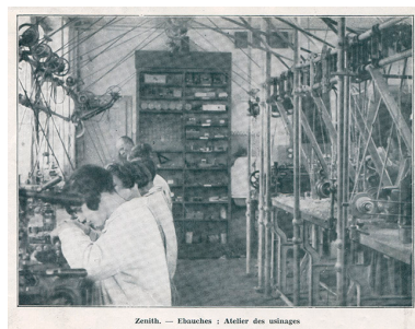
Zénith. - Ebauches : atelier des usinages, 1933. IVR43_20162500579NUC2A
