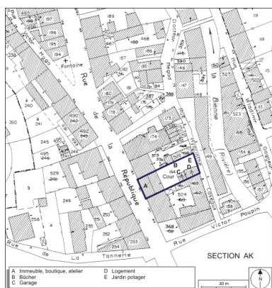
Plan-masse et de situation. Extrait du plan cadastral, 1980, section AI, échelle 1:1000. Dess. André Céréza IVR43_20093900304NUDA
