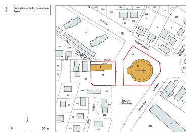
Plan masse et de situation, extrait cadastral de la Direction Générale des Finances Publiques (DGFIP) 2022, échelle 1/1000e. Dess. Aline Thomas IVR26_20258900140NUDA
