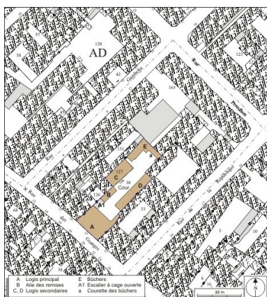
Plan masse et de situation. Extrait du plan cadastral, 1974, section AD. Dess. André Céréza IVR43_20102500064NUDA
