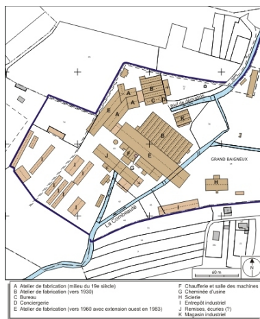
Plan-masse et de situation. Extrait du plan cadastral numérisé,
