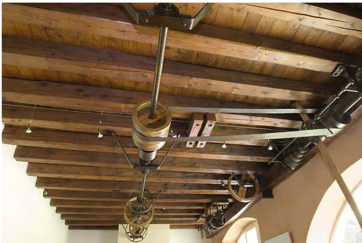
Usine : transmission au plafond.
