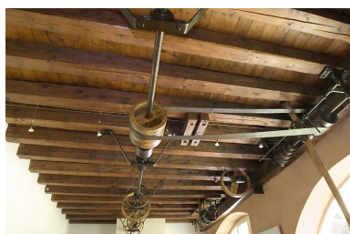
Usine : transmission au plafond. Phot. Jérôme Mongreville IVR43_20082501133NUC2A
