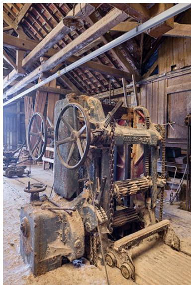
Châssis multilames vu de trois quarts arrière. Phot. Jérôme Mongreville IVR43_20162500430NUC4A
