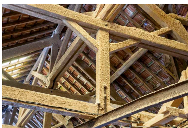
Détail de la charpente de l'atelier. Phot. Jérôme Mongreville IVR43_20162500437NUC4A
