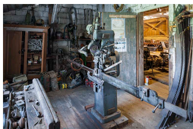
Atelier d'affûtage. Phot. Jérôme Mongreville IVR43_20162500439NUC4A
