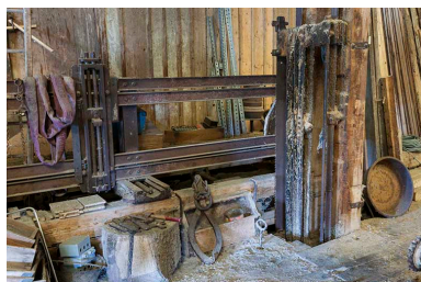
Châssis vertical monolame dit "sabre". Phot. Jérôme Mongreville IVR43_20162500438NUC4A
