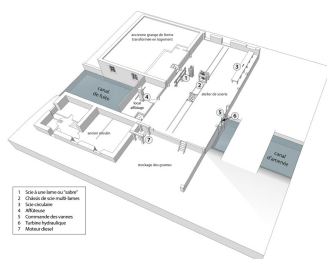
Schéma en 3D avec disposition des machines. Dess. Mathias Papigny IVR43_20162501770NUDAQ
