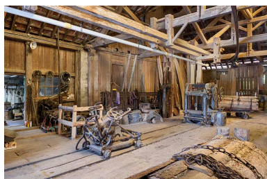
Vue d'ensemble de l'atelier de scierie. Phot. Jérôme Mongreville IVR43_20162500427NUC4A
