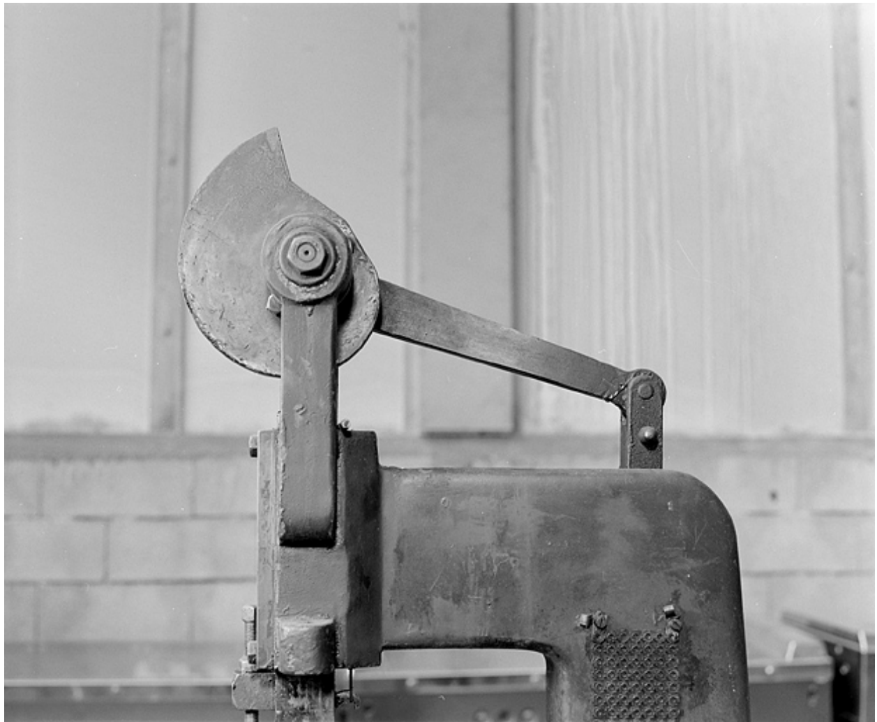
Vue de profil de la came.
