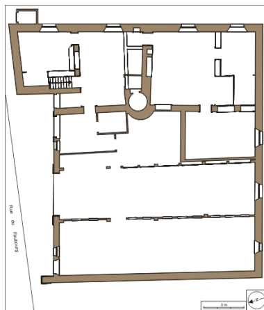
Plan au sol. Dess. André Céréza IVR43_20092501587NUDA
