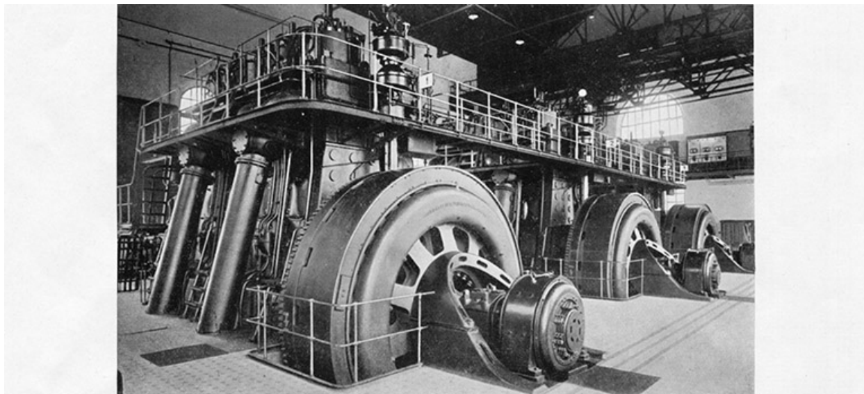
STATION DE SECOURS D'ÉTUPES : Salle des machines comprenant 3 groupes Diesel-alternateur de 1.500 CV chacun.
