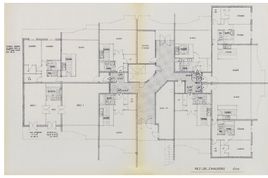
Opération de 132 logements : plan du rez-de-chaussée des immeubles ; F. Martin Lavigne, D. Chenut, O. Senly, septembre 1979. (Archives municipales Cosne-Cours-sur-Loire, 200 W 115 - PC 684) Phot. Thierry Kuntz, Autr. F. Martin Lavigne, Autr. D. Chenut, Autr. O. Senly IVR26_20145800191NUC2A
