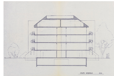
Opération de 132 logements : coupe générale des immeubles ; F. Martin Lavigne, D. Chenut, O. Senly, septembre 1979. (Archives municipales Cosne-Cours-sur-Loire, 200 W 115 - PC 684) Phot. Thierry Kuntz, Autr. F. Martin Lavigne, Autr. D. Chenut, Autr. O. Senly IVR26_20145800196NUC2A
