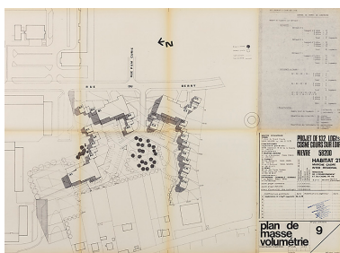
Opération de 132 logements : plan de masse et volumétrie ;
