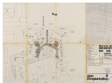
Opération de 132 logements : plan d'implantation ; F. Martin Lavigne,
