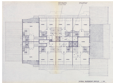
Opération de 132 logements : plan du dernier étage des duplex des immeubles ; F. Martin Lavigne, D. Chenut, O. Senly, septembre 1979. (Archives municipales Cosne-Cours-sur-Loire, 200 W 115 - PC 684) Phot. Thierry Kuntz, Autr. F. Martin Lavigne, Autr. D. Chenut, Autr. O. Senly IVR26_20145800195NUC2A
