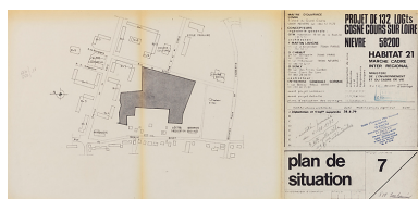
Opération de 132 logements : plan de situation ; F. Martin Lavigne, D. Chenut, O. Senly, août 1979.
