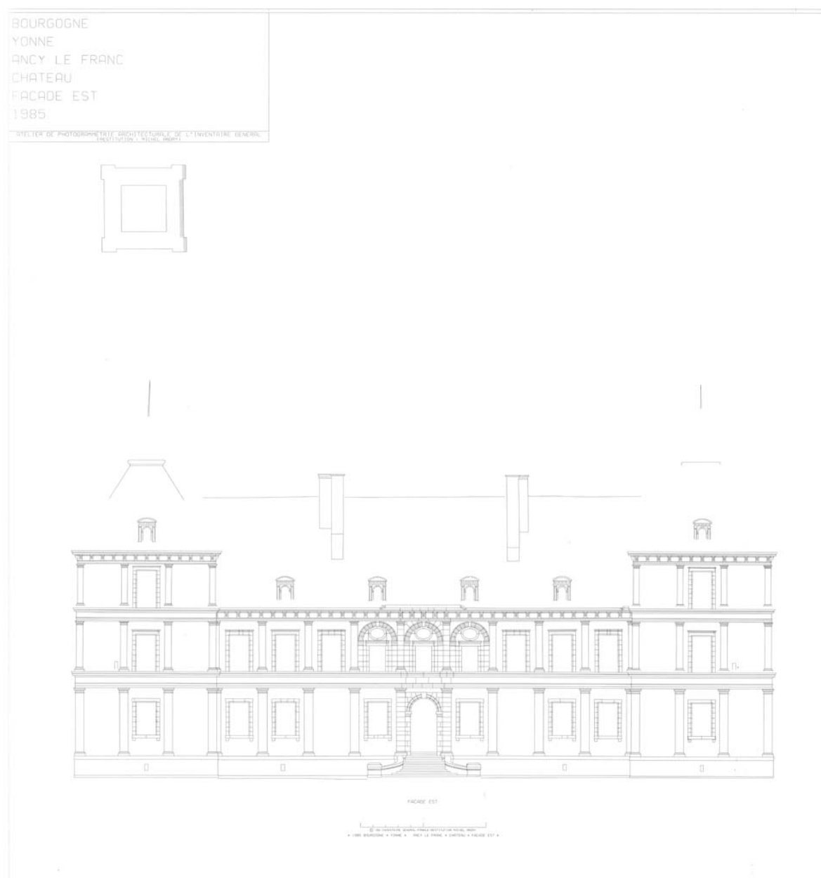
Façade est, restitution photogrammétrique.
