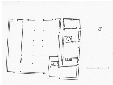
Plan au sol. Phot. Dominique et Sancey Dominguez IVR43_19792500010V
