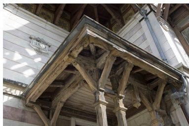
Elévation antérieure : charpente du porche. Phot. Yves Sancey IVR43_20093900158NUC2A
