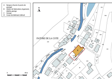
Plan-masse et de situation. Extrait du plan cadastral, 2017, section AC, 1/1 000. Dess. Mathias Papigny IVR43_20172501255NUDA
