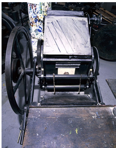
Vue de détail plongeante. Du premier au dernier plan : table de marge, platine et ses raquettes, rouleaux encres, marbre équipé d'un dispositif d'emporte-pièce (pour réaliser de la découpe), table d'encrage et soleil. Phot. Jérôme Mongreville IVR43_20013900762XA
