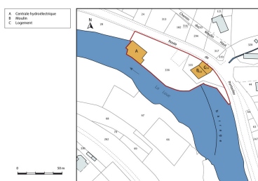
Plan-masse et de situation. Extrait du plan cadastral, 2016, section AC. Dess. Mathias Papigny IVR43_20162501759NUDA
